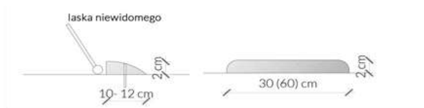
Rys. D3 – Profil rozdzielający ruch rowerowy od pieszego. Sygnalizujący koniec ciągu pieszego
